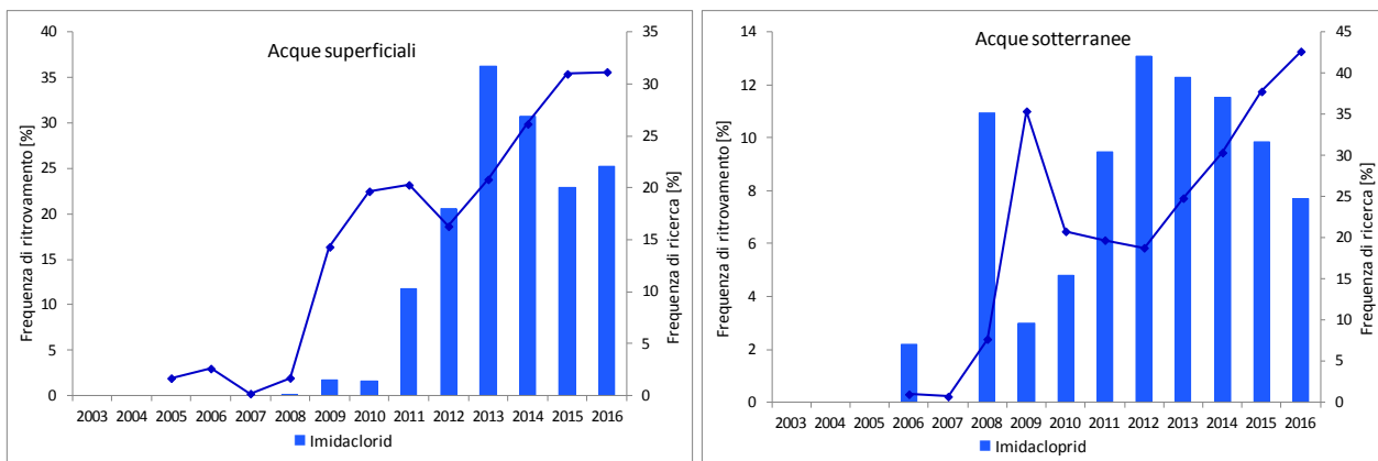
Fig. 9.18 – Trend dell'imidacloprid
